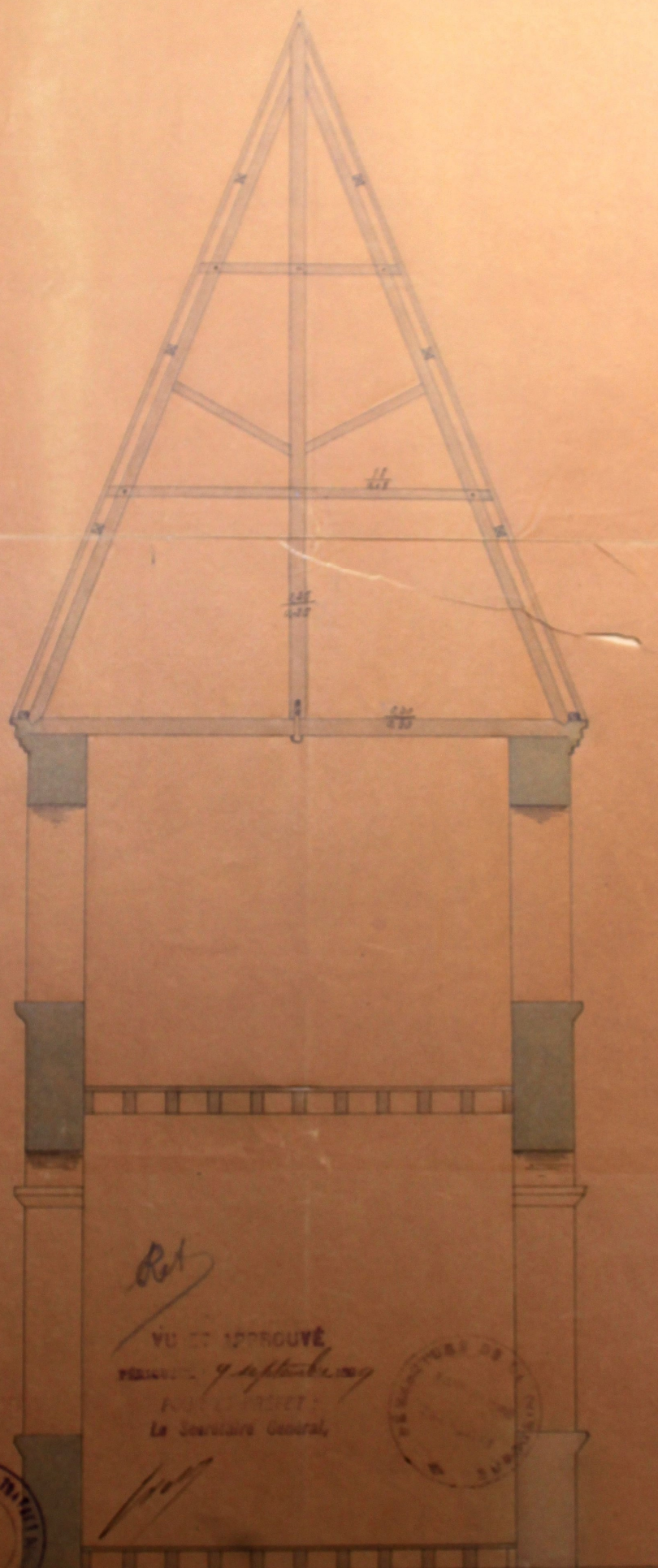
Coupe du clocher à partir de l'extrados des voûtes
