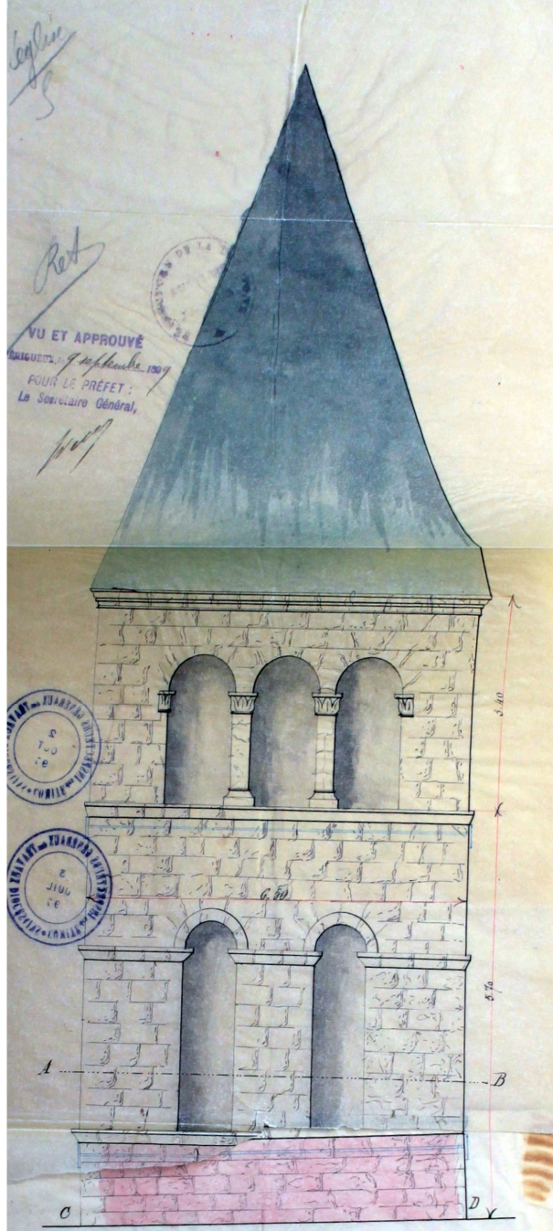
Élévation à partir de l'extrados des Toites
